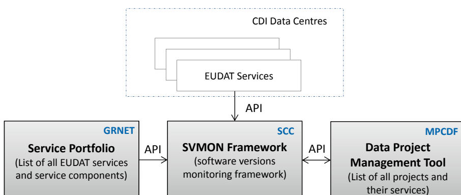
Abb. 2: Schema der automatisierten Software-Versions-Überwachung innerhalb der CDI.
